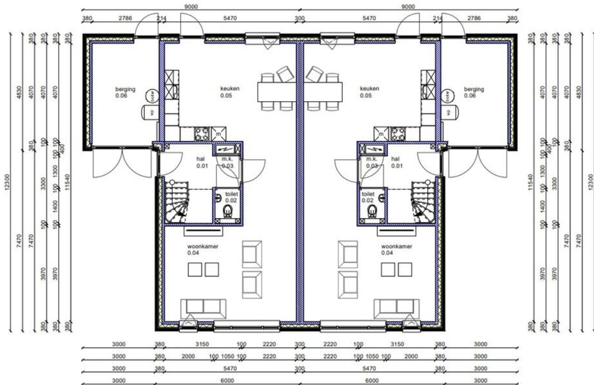
Begane grond
