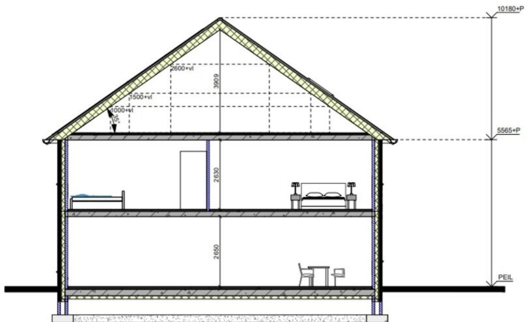
Doorsnede
