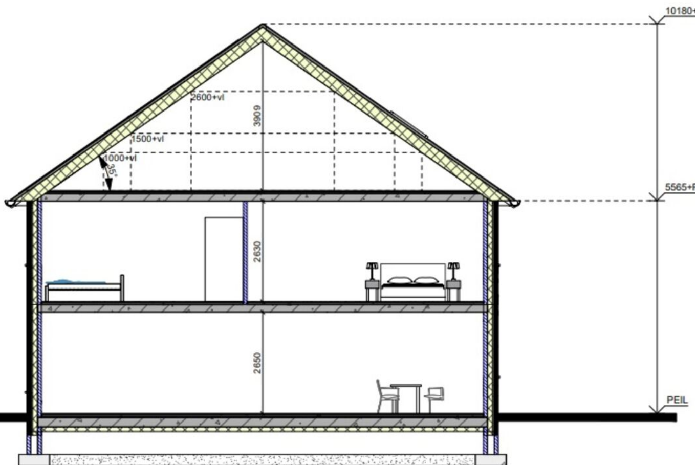
Doorsnede
