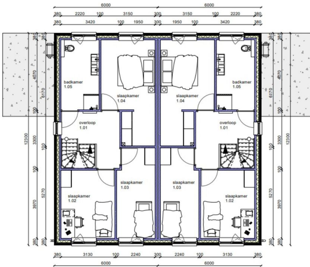
Verdieping
